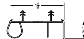
EVERLAST SWEEP
