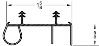
EVERLAST SWEEP - PVC WS-025
