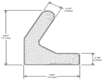
WS-016 Double Door Astragal (August 2015 - Current)
