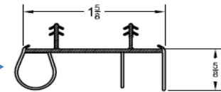
EVERLAST SWEEP WS-006E
