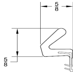
WS-011 Compression Jamb Kerf Seal
