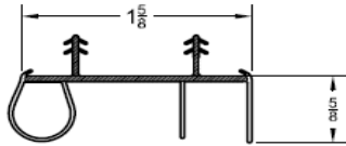
EVERLAST SWEEP WS-006E
